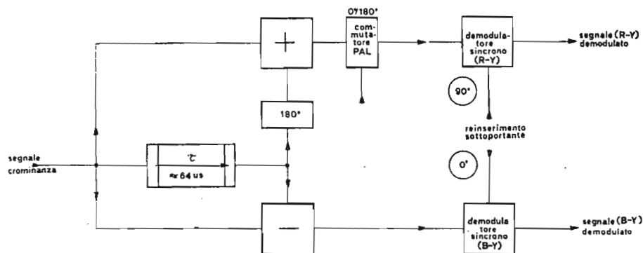
Fig. 2 - Schema a blocchi di un demodulatore PAL. Il segnale di crominanza a 4,43 MHz diretto e ritardato viene contemporaneamente sommato (+) e sottratto (-) nella matrice PAL della linea di ritardo, per cui all'uscita dello stadio somma di detta matrice avremo il segnale (R—Y) a 4,43 MHz mentre all'uscita dello stadio differenza avremo il segnale (B—Y) a 4,43 MHz. L'alternanza caratteristica del segnale (R—Y) può essere tolta da un apposito commutatore e all'atto della sua demodulazione sia prima della demodulazione (come è il caso in questo schema). Per demodulare i segnali differenza di colore (R—Y) e (B—Y) a 4,43 MHz occorre reinserire la portante soppressa in trasmissione, ciò ha luogo nei due demodulatori sincroni di detti segnali. La frequenza e la fase di questa portante rigenerata nel televisore viene controllata dal « burst » dal quale vengono anche ricavati i segnali di identificazione per il pilotaggio del commutatore PAL.
